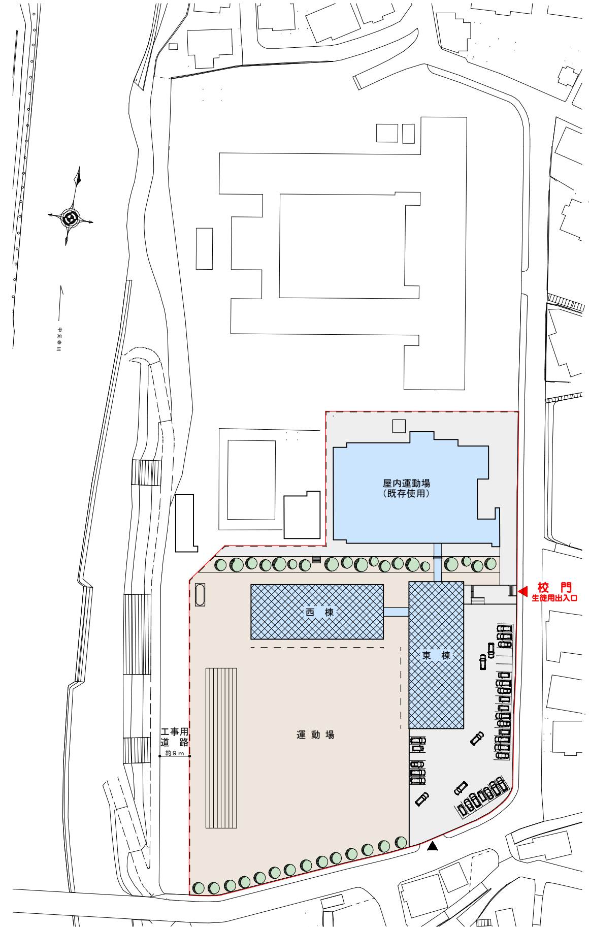
後藤寺中学校 仮設校舎配置図
